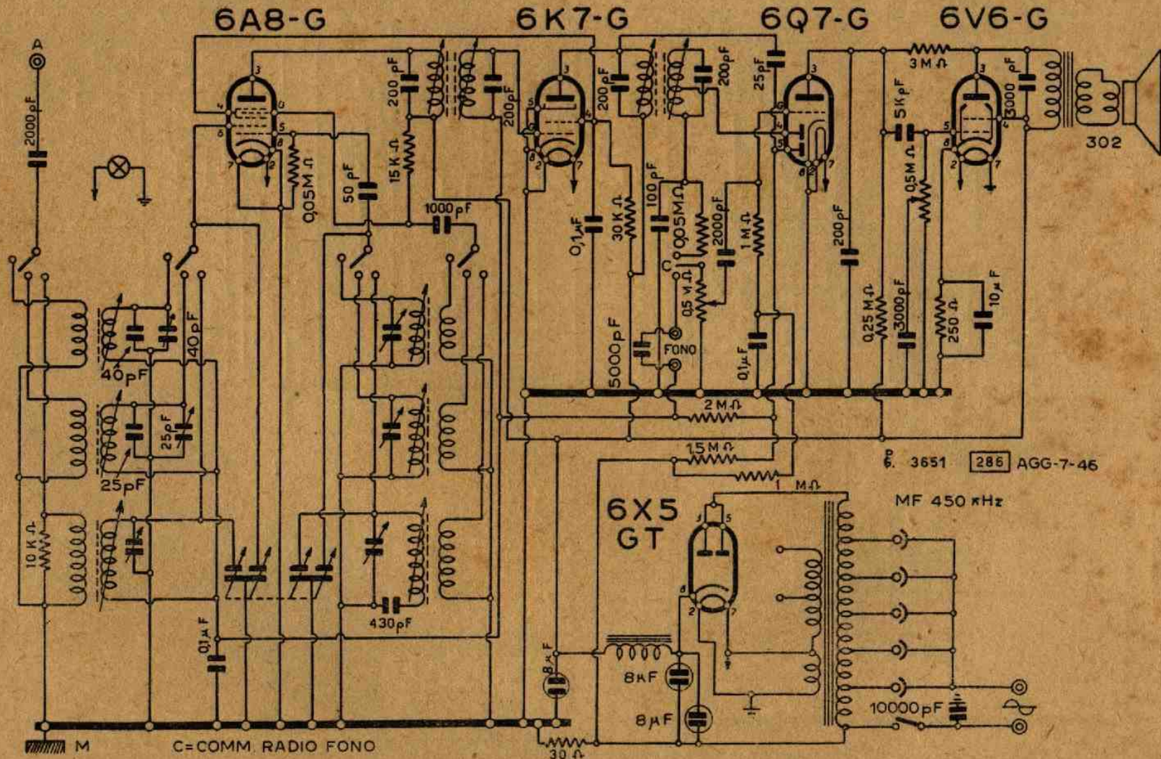
Lo schema elettrico del Tri-Unda R 53/4
